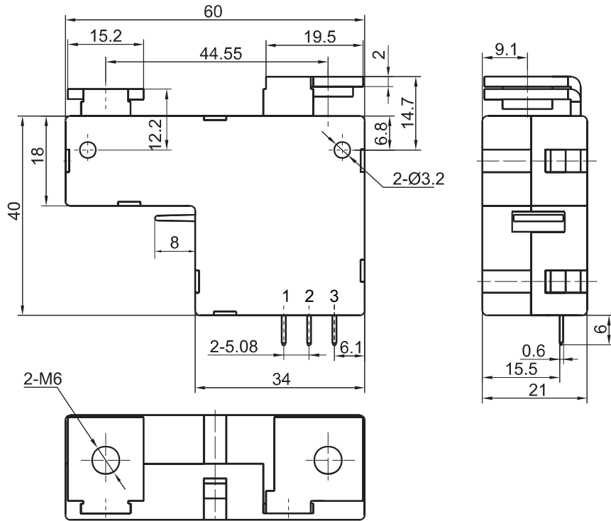
Outline Dimensions 外形图
